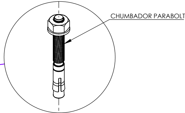
DETALHE C ESCALA 1 : 2
