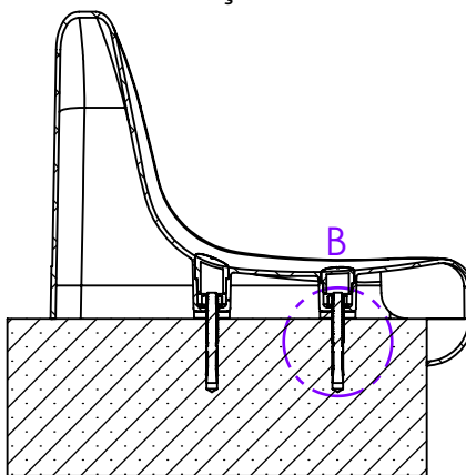
SEÇÃO A-A
