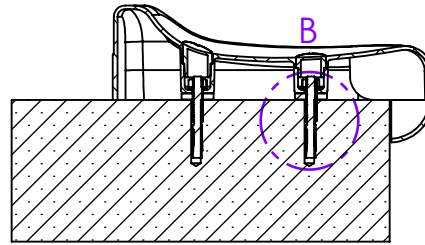
SEÇÃO A-A
