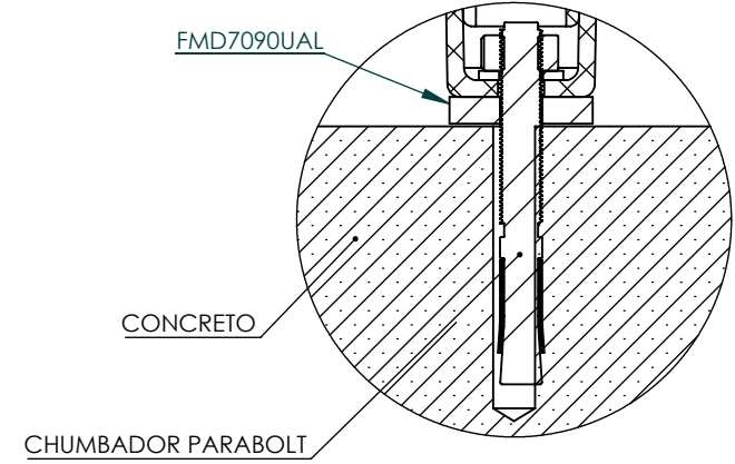
DETALHE B ESCALA 1 : 2
