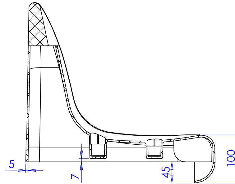
SEÇÃO B-B
