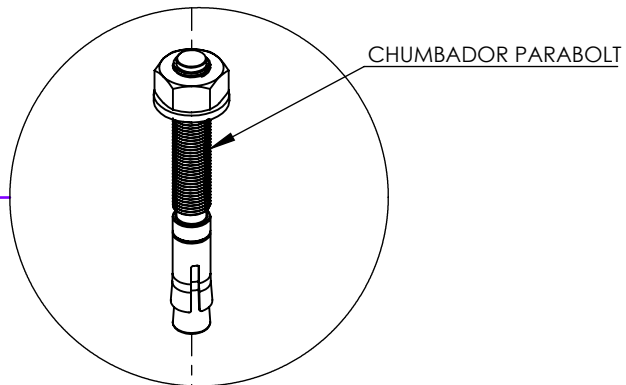
DETALHE C ESCALA 1 : 2
